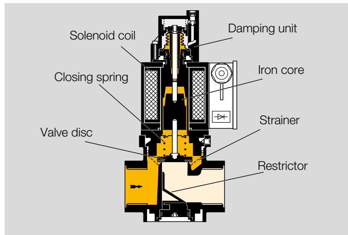
VG 15–40/32..R..L
