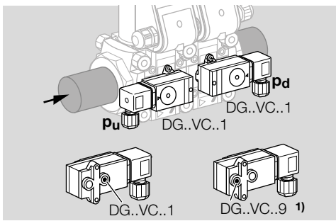
1) DG..VC..9 для последующего монтажа
